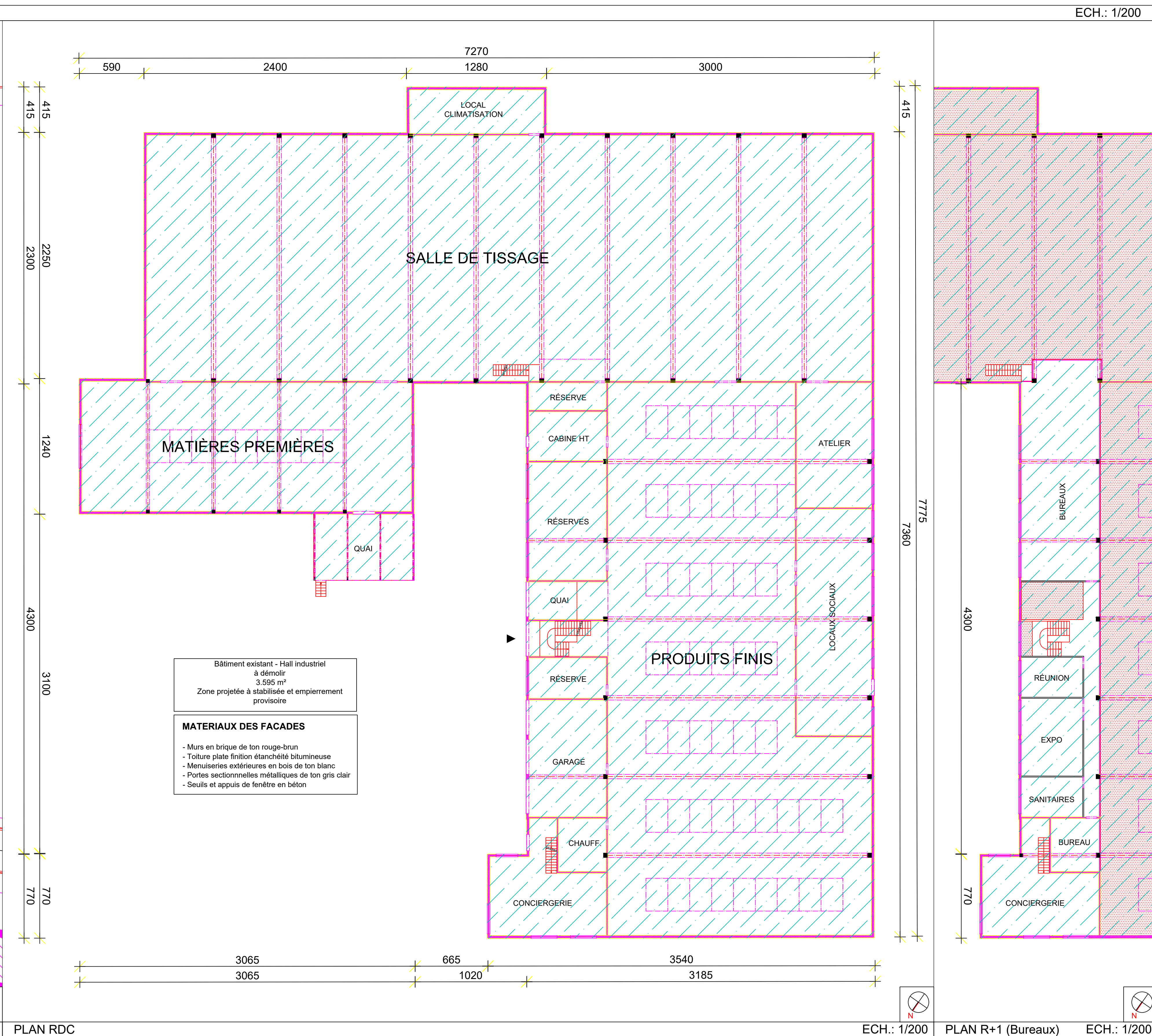
PLAN RDC ECH.: 1/200
