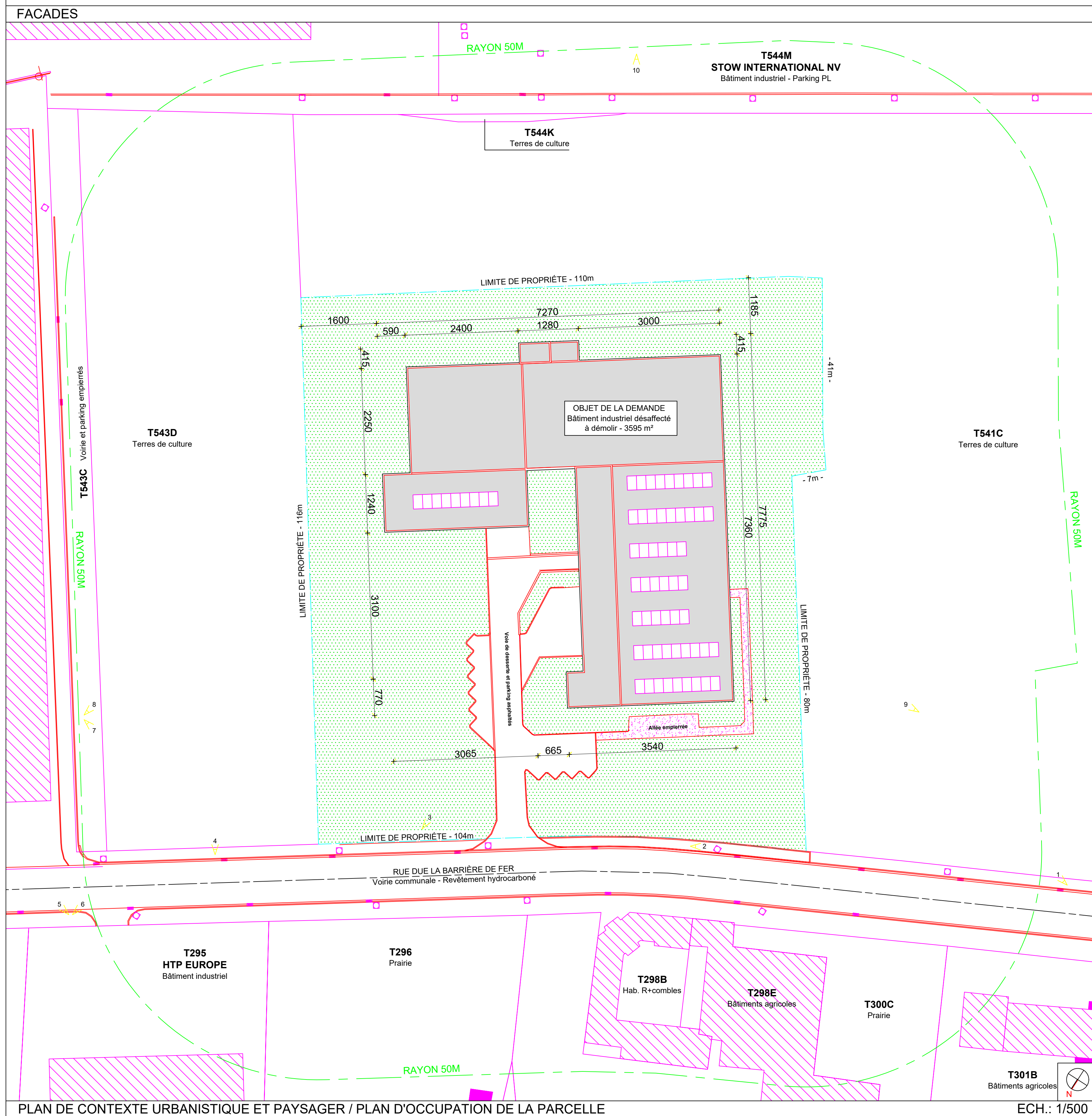
PLAN DE CONTEXTE URBANISTIQUE ET PAYSAGER / PLAN D'OCCUPATION DE LA PARCELLE ECH.: 1/500
